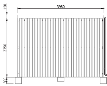
FalcoLok-600VH, 1 modul, med enkeltdør DIN-højre og hårdtræbeklædning
