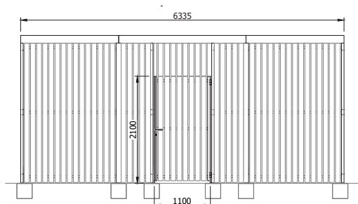
FalcoLok-600VH, 1 modul, med enkeltdør DIN-højre og hårdtræbeklædning
